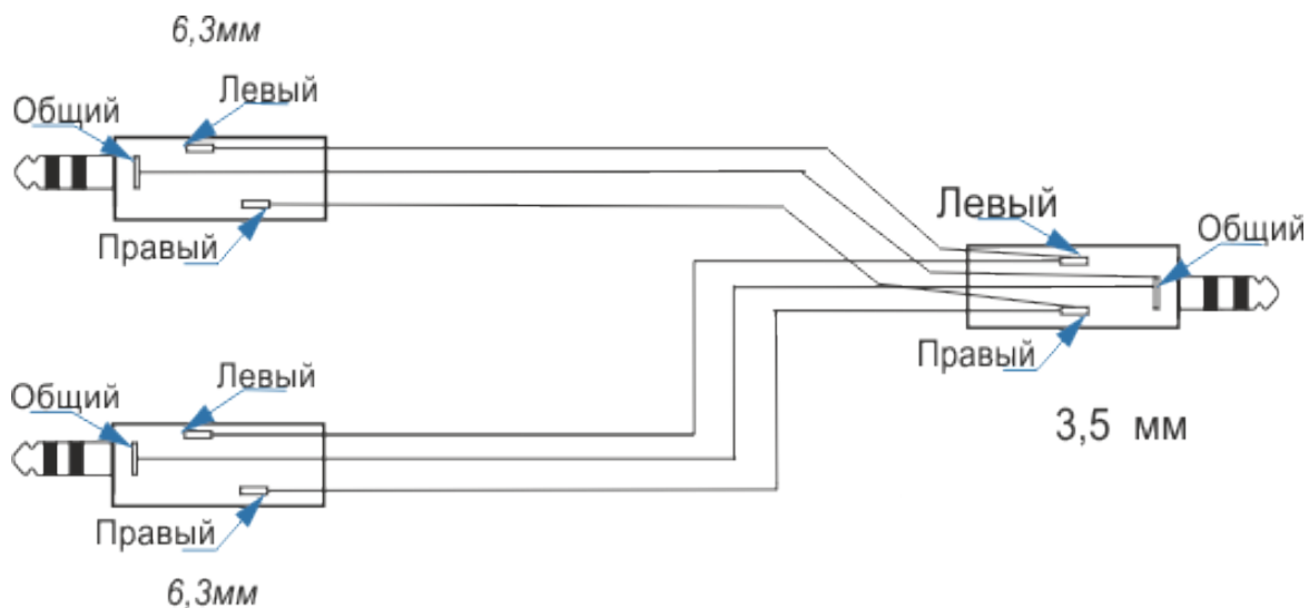
Рисунок 7 - Схема разводки аудио кабеля для связи «Тромбон БЧС-М» с прибором управления «Тромбон ПУ-ХХ»
