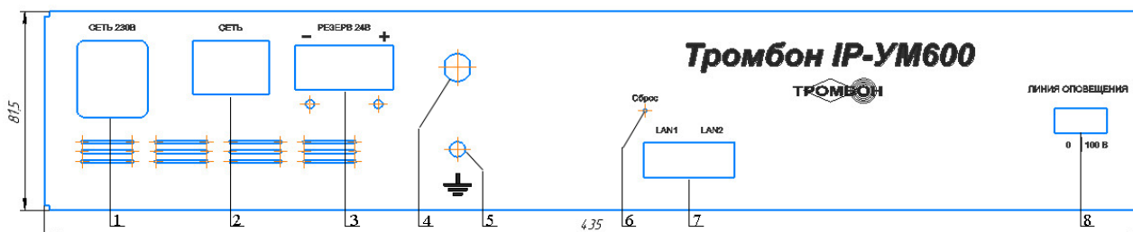
Рисунок 2 - Вид сзади
